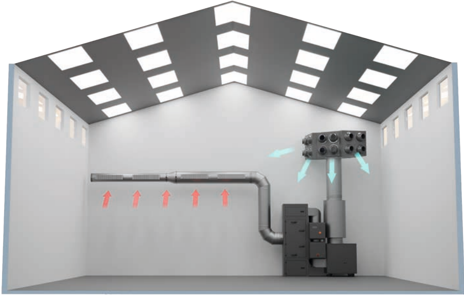
Kurulum örneği: BlowTec sistemi bir salonda
