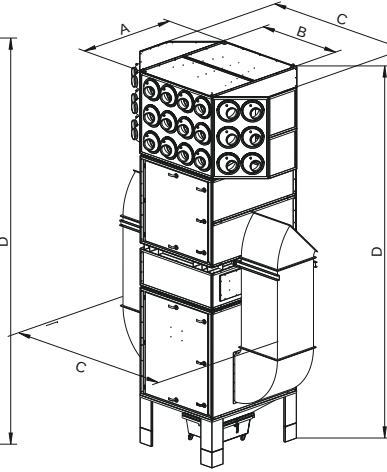
Ses yalıtım gövdesiz tesis
