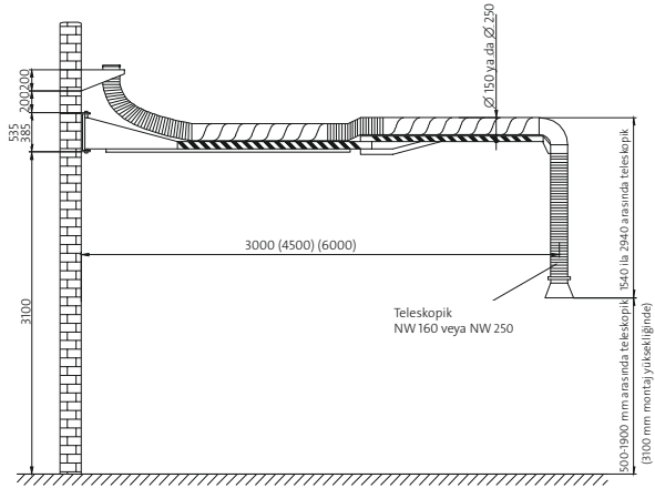
Emme vinci (ürün no. 97 641)
