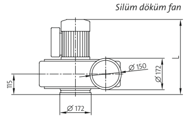
Silüm döküm fan
