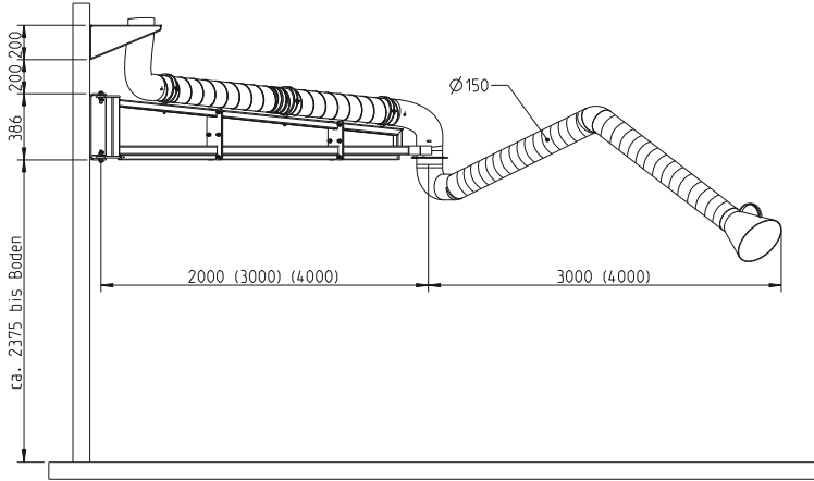
Duvar kollu ve kılavuz raylı emme kolu
