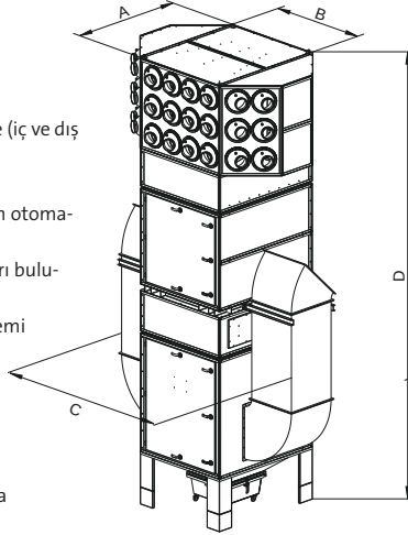
Ses yalıtım gövdeli tesis
