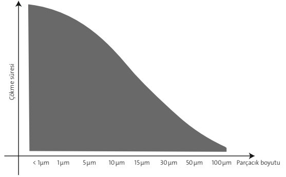
Diyagram: Parçacıklar ne kadar küçükse, o kadar yavaş çökeltirler
