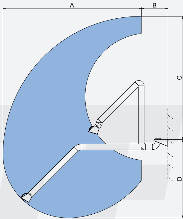
Abb. Absaugarm mit Erfassungsradius in Seitenansicht
