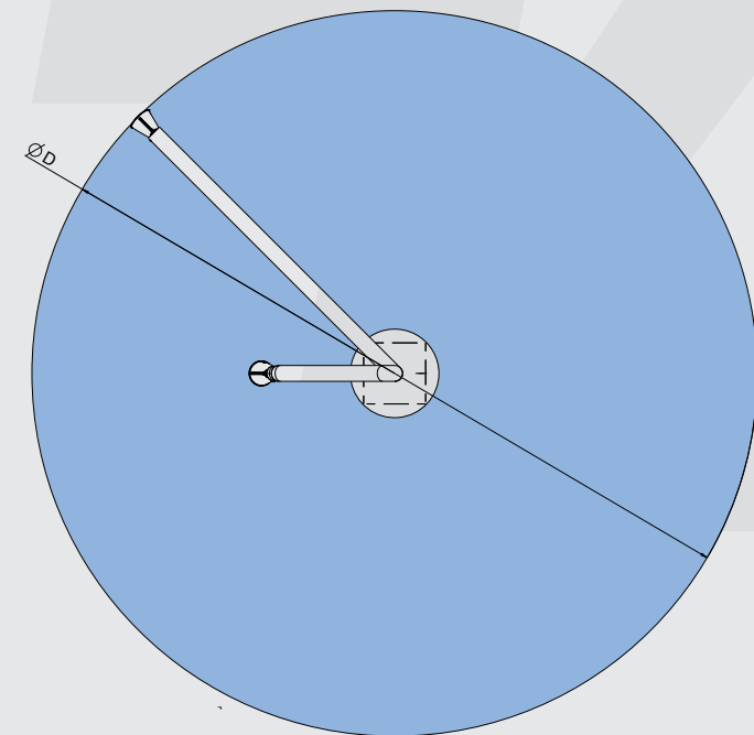
Abb. Absaugarm mit Erfassungsradius in Draufsicht
