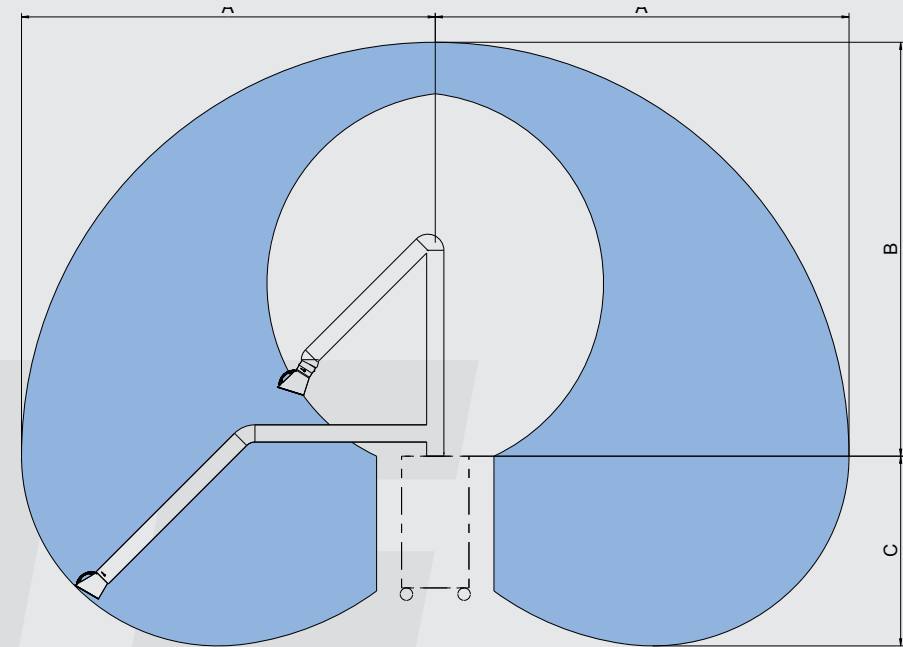
Abb. Absaugarm mit Erfassungsradius in Seitenansicht
