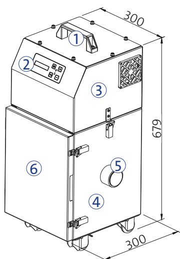
Diseño sin limpieza automática
