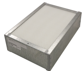
Filtro Ulpa U16, dimensiones: 337 x 230 x 100 mm Producto No.: 100350005
